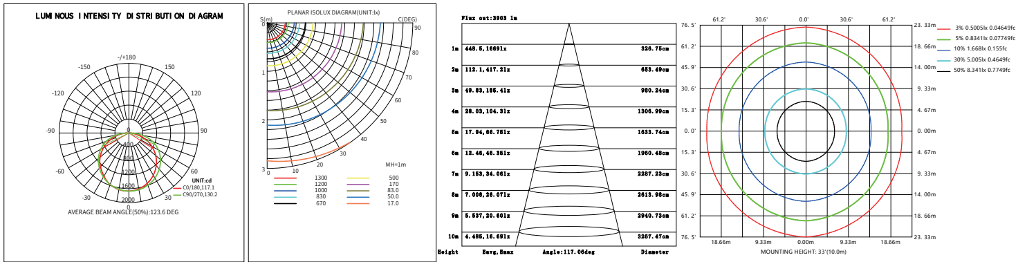
CL-TRF14-TCP40W-CCT (@ 40W @ 5000K)
