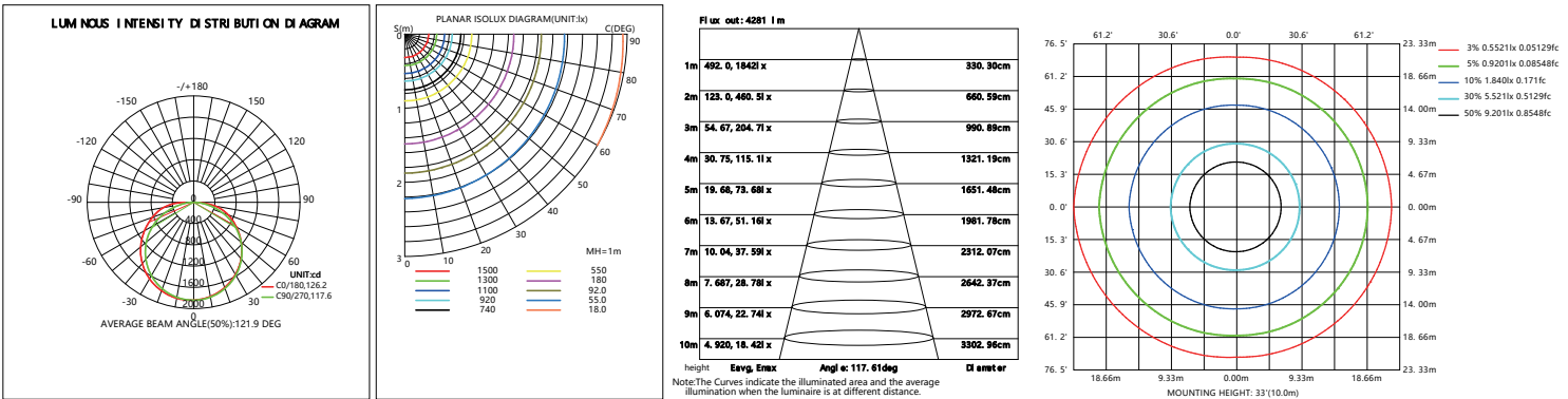
CL-TRF22-TCP40W-CCT (@ 40W @ 5000K)
